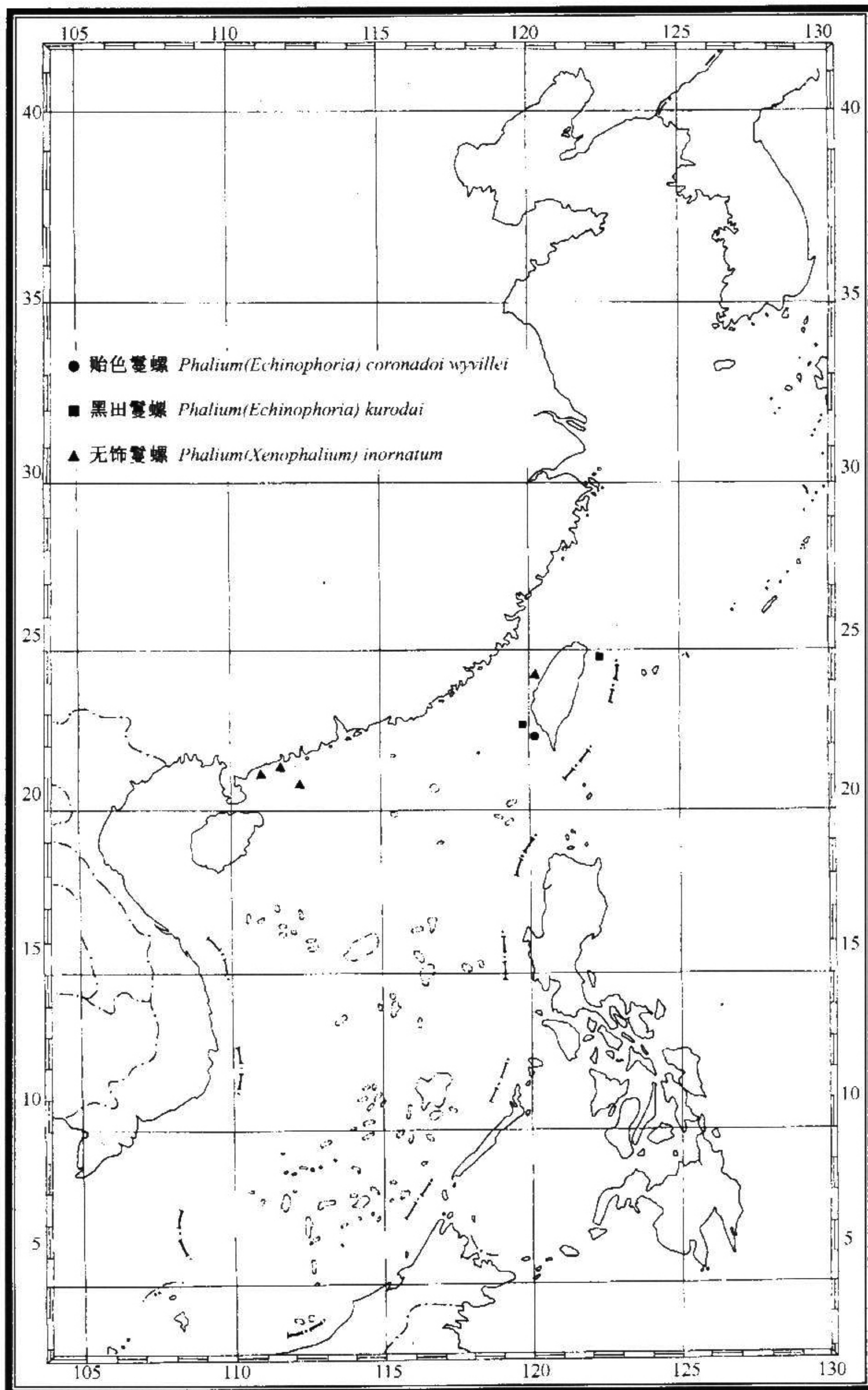
图 30 冠螺科种类在中国近海的分布 (5)
